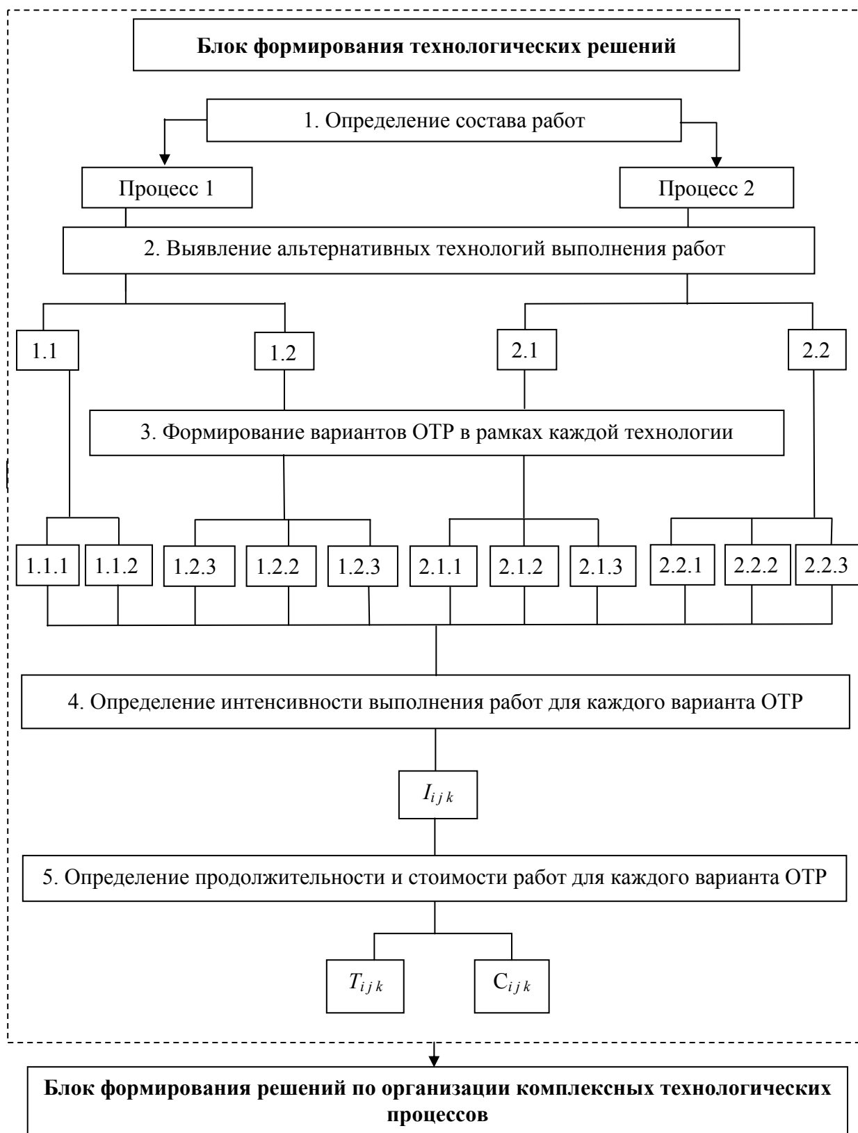
Рис. 3.2. Последовательность формирования ОТР выполнения строительных работ на вариантной основе: I_{ijk} — интенсивность осуществления i -го строительного процесса для j -й технологии для k -го варианта организационно-технологического решения его выполнения (по составу задействованных ресурсов); T_{ijk} — продолжительность осуществления i -го строительного процесса для j -й технологии для k -го варианта его выполнения; C_{ijk} — прямые расходы на осуществление i -го строительного процесса для j -й технологии для k -го варианта его выполнения
