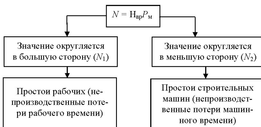
Рис. 3.3. Варианты формирования технологической системы «машина(ы) — рабочие»
